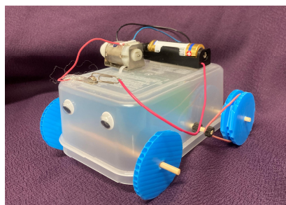
図 お掃除ロボット完成予想
