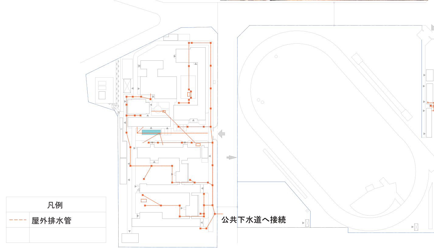
排水中継槽
