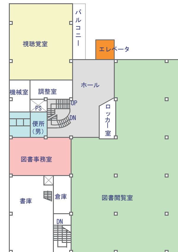
図書館2階平面図
