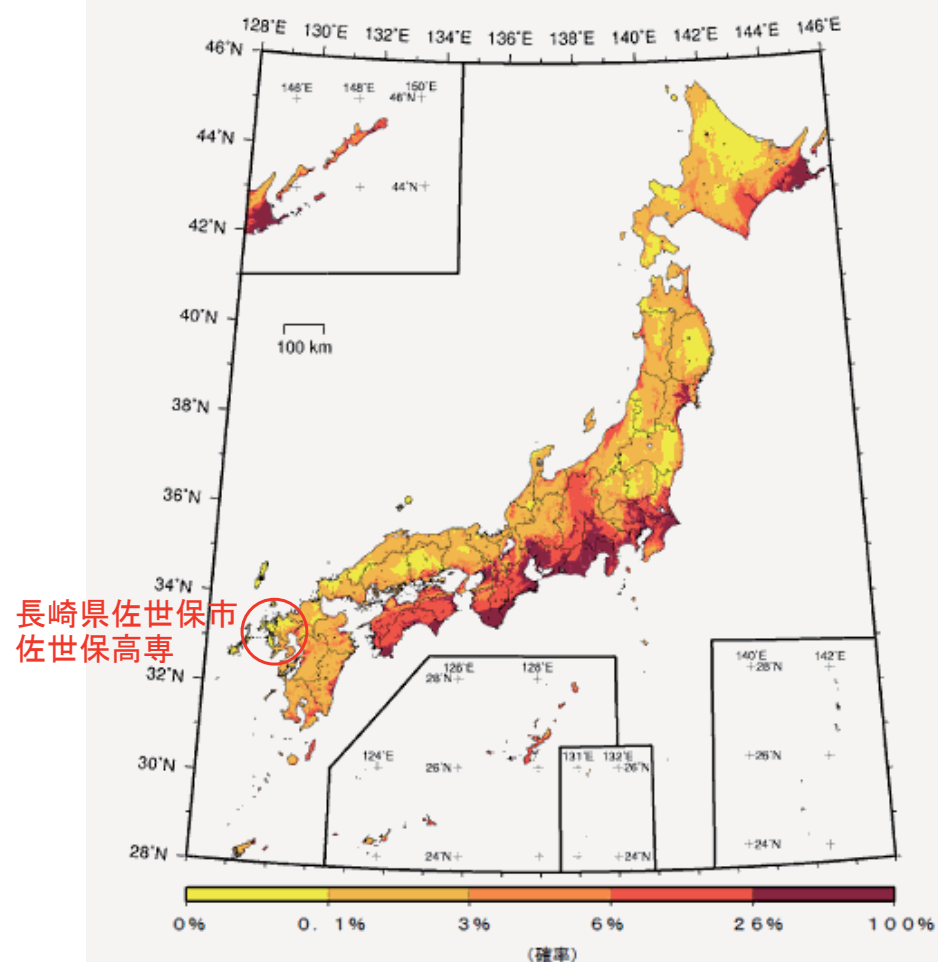
確率論的地震動予測地図
