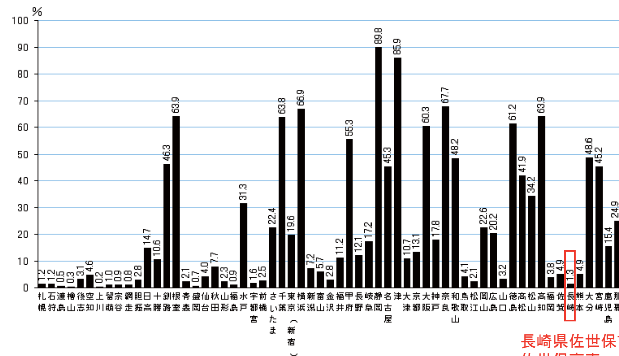
地域別の大地震発生確率(2010年)
