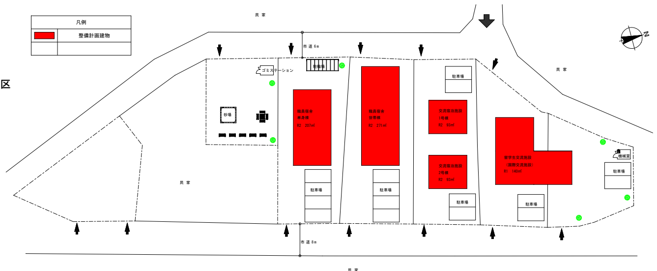
整備計画 配置図 S=1/500
