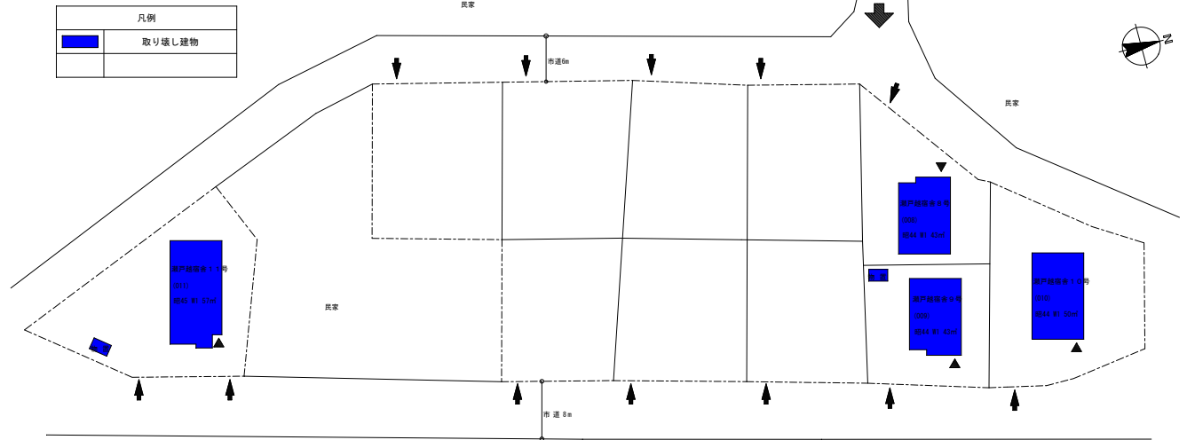
既設 配置図 S=1/500
