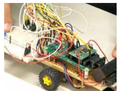
工学実験・実習 (マイコンカー製作) Electrnic Experiments (Micom Car)
