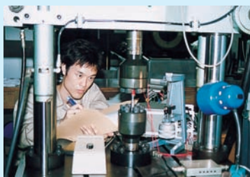
引張り圧縮疲労試験 Serbopulser
